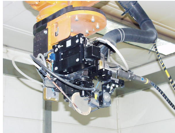
AFO 210 – laserová hlava
