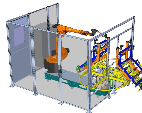
3D návrh pracoviště
