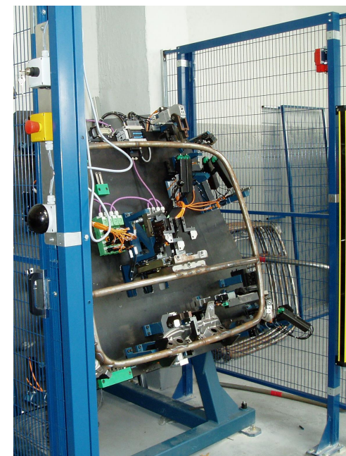
Měřicí přípravek
