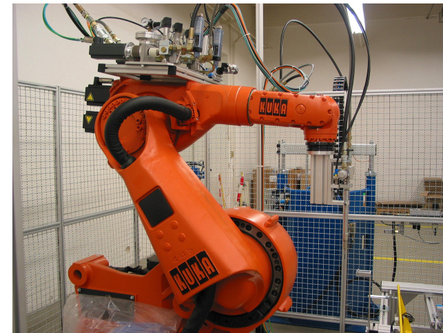
Kleben Zuführeinheit
