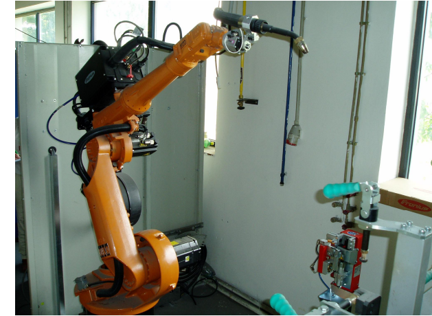
Schweißtesten mit TIG-Methode
