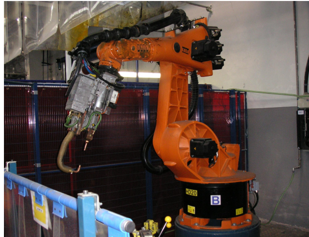
Schweißroboter B
