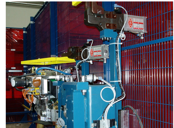
Schneller Austausch von Schweißzangen
