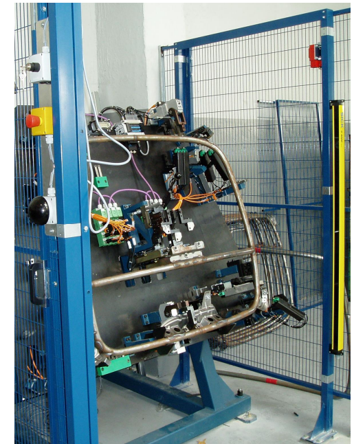
Festspannende Vorrichtung
