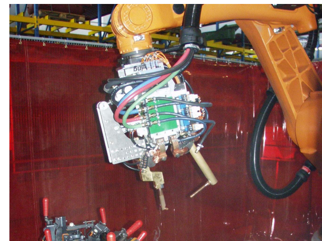
Сварочные клещи
