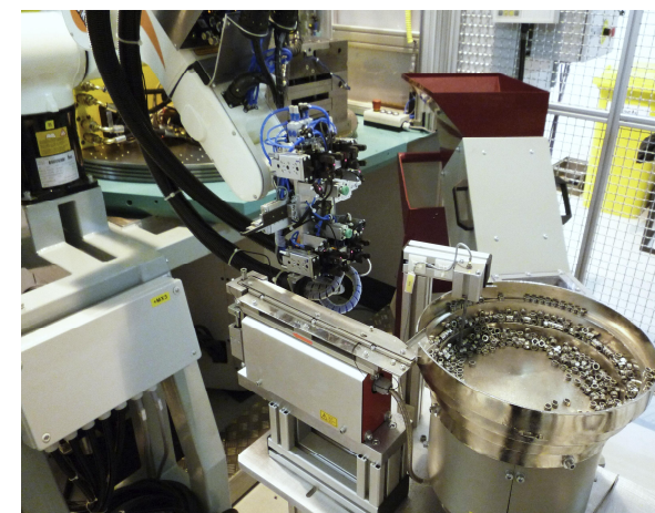
Щупальце робота В и вибрационный питатель
