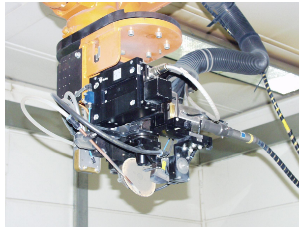
AFO 210 – голова лазера
