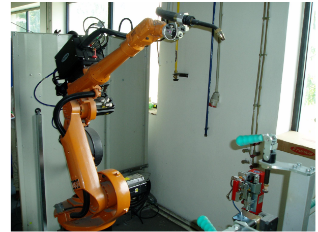
Тестирование сварки методом TIG
