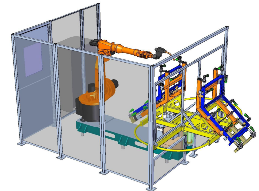
3D дизайн рабочего места
