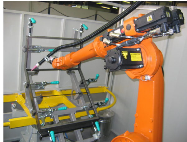
Установка кармушки и факеля MIG
