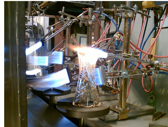
Выход из полировщика
