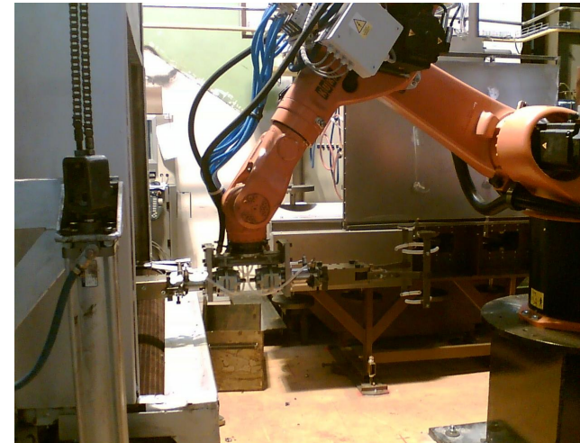
Робот перед печей переохлаждения
