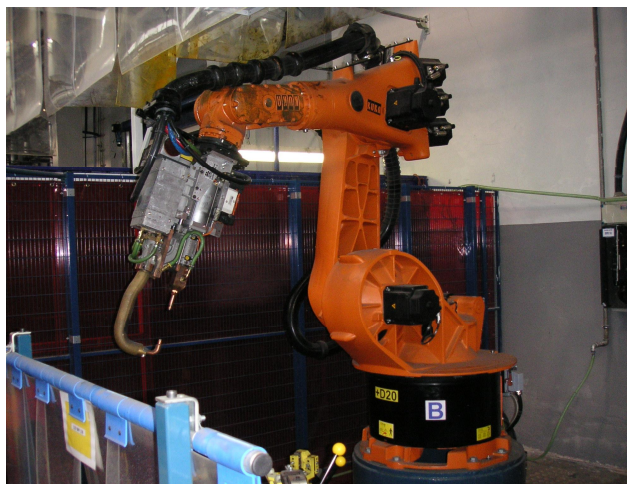
Сварочный робот Б
