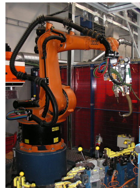
Сварочный робот А
