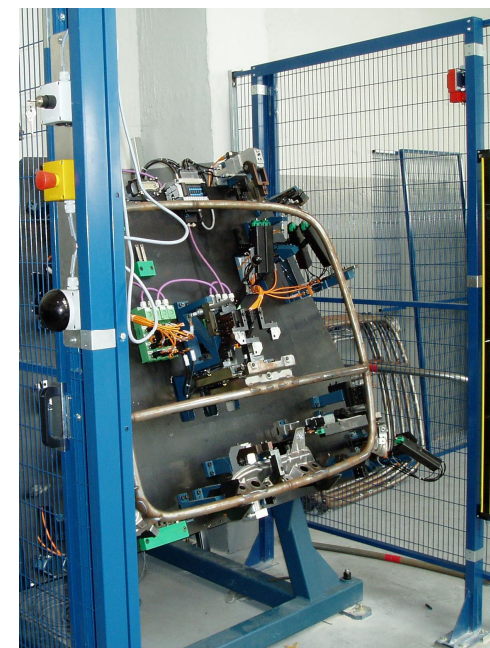
Мерительное приспособление
