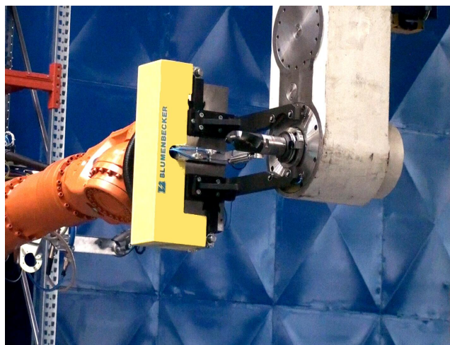
Загрузка инструмента в шпиндель обрабатывающего центра
